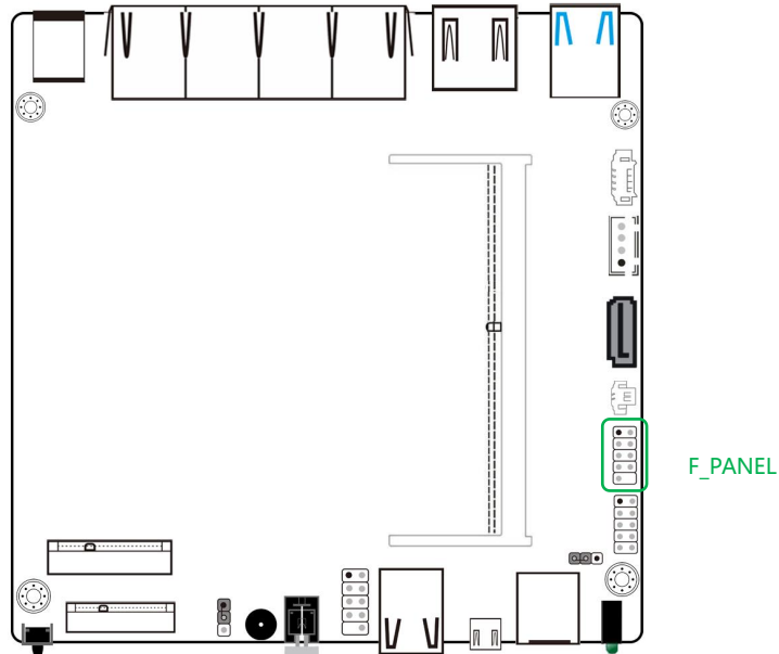
F_PANEL (2×5 pin 间距 2.54mm 第 10 pin 空)
