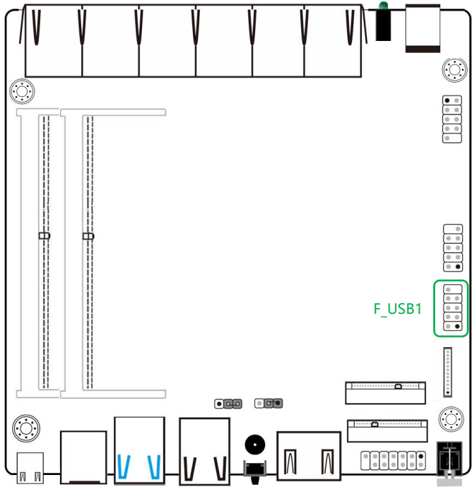
F_USB1 (2×5 pin 间距 2.54mm 第 9 pin 空)
